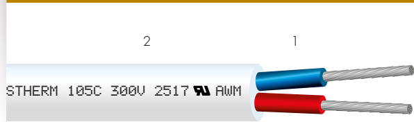
1 • Conductores de aislamiento PVC homologados UL y cUL. 2 • Cubierta exterior: PVC.
