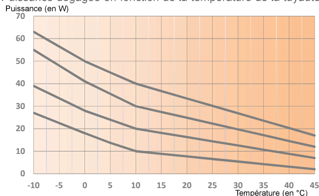
Puissance dégagée en fonction de la température de la tuyauterie
