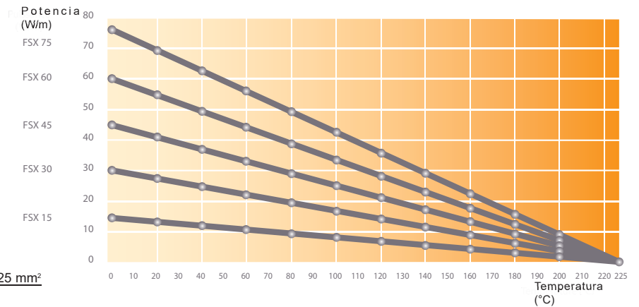
Potencia liberada en función de la temperatura de la tubería
