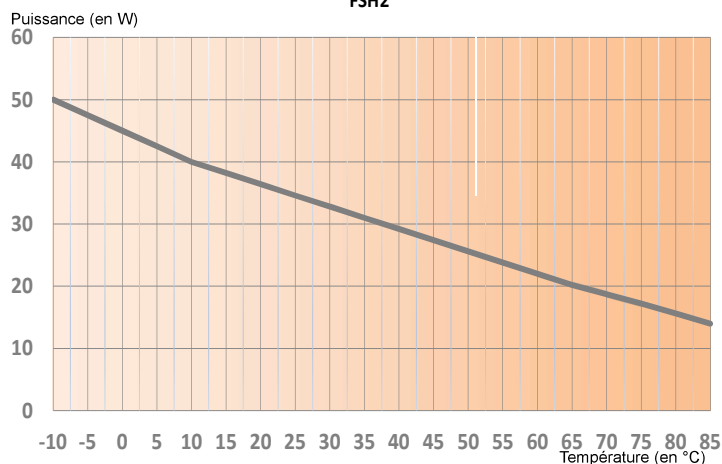
Puissance dégagée en fonction de la température de la tuyauterie FSH2
