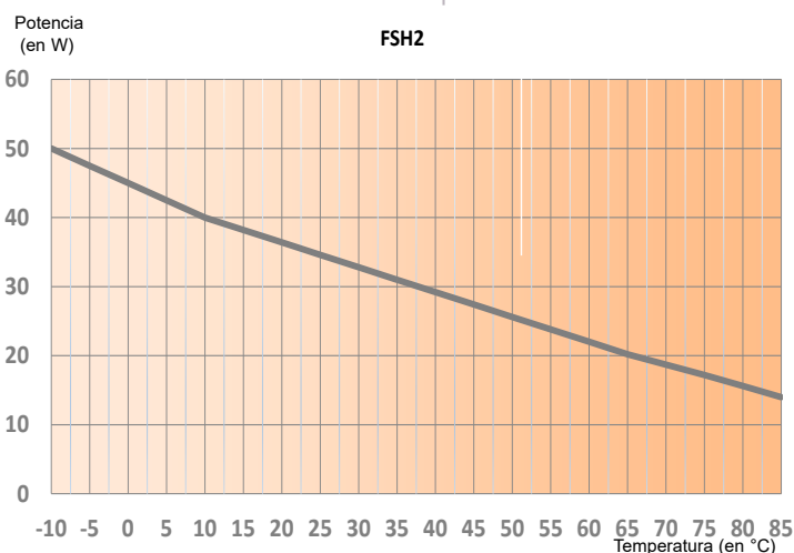
Potencia liberada en función de la temperatura de la tubería
