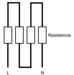
Ejemplo de alambrado eléctrico tipo 2
