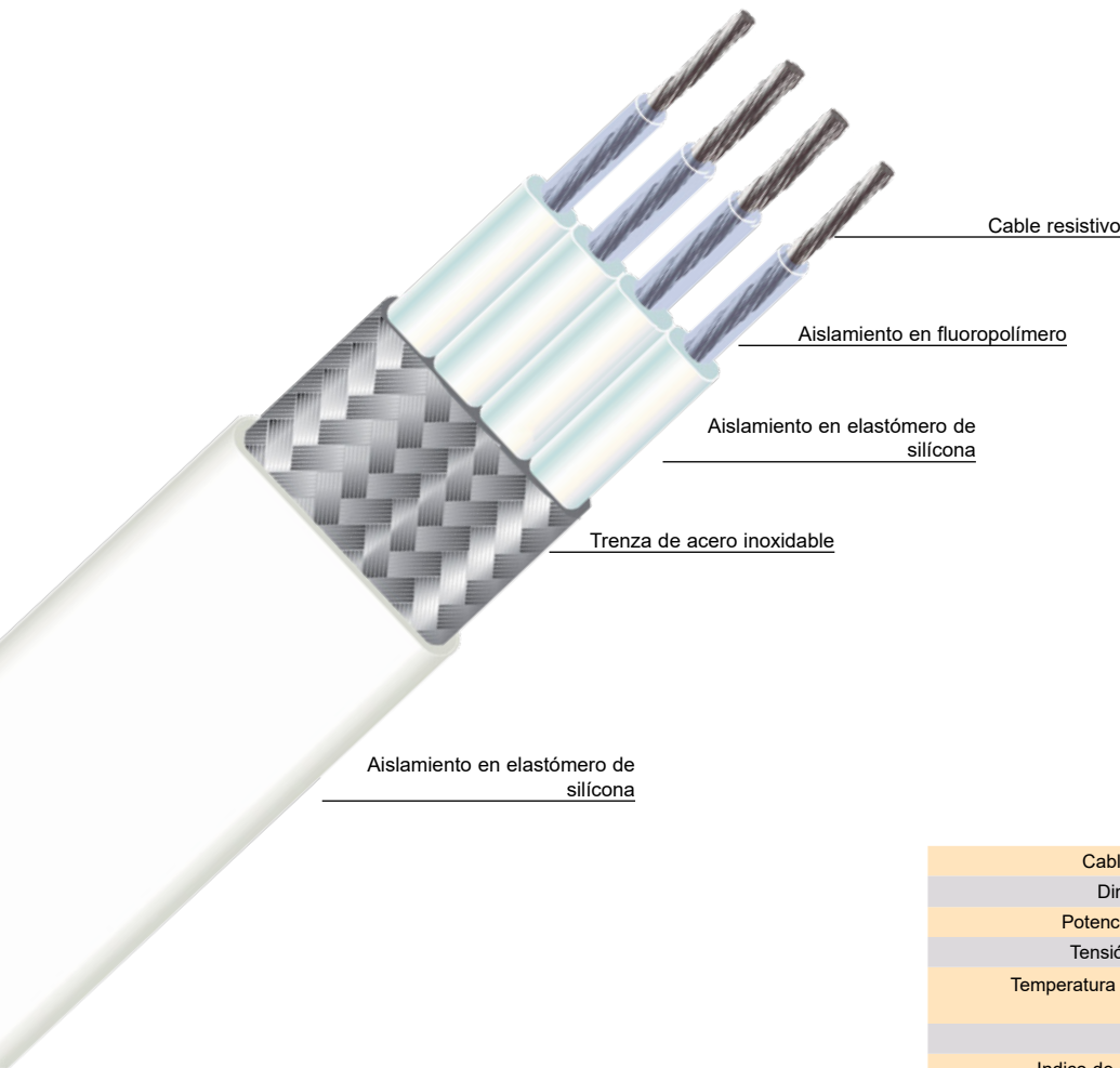
Ejemplo de alambrado eléctrico tipo 2
