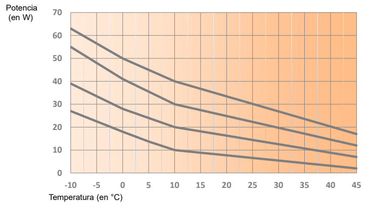
Potencia liberada en función de la temperatura de la tubería
